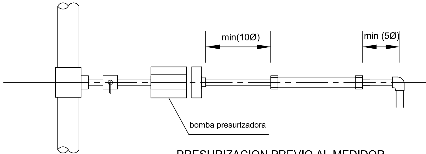
PRESURIZACION PREVIO AL MEDIDOR
